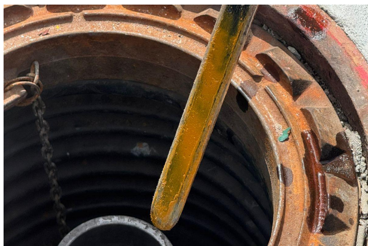
MEDICIÓN Y CORTE DE AGUA LIBRE EN LOS TANQUES DE ALMACENAMIENTO
